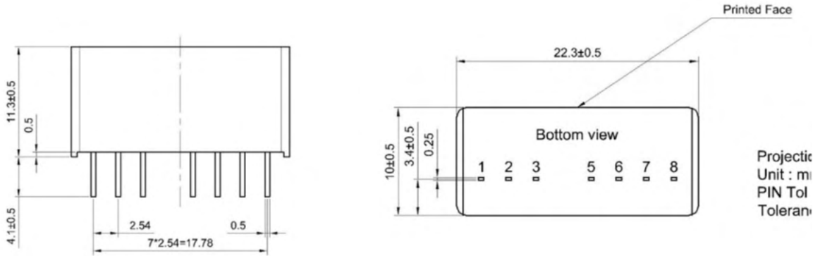
ピン配置
