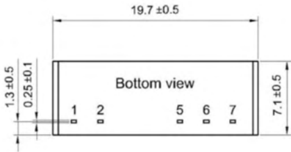
ピン配置
